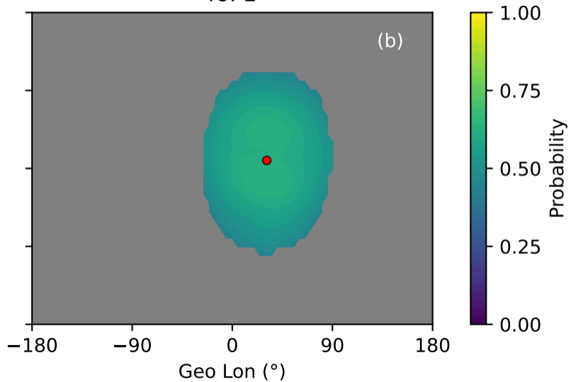
foF1
